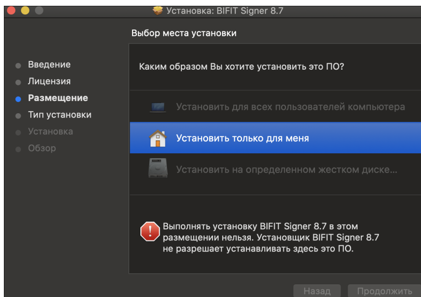
Рис. 10. Выбор размещения
