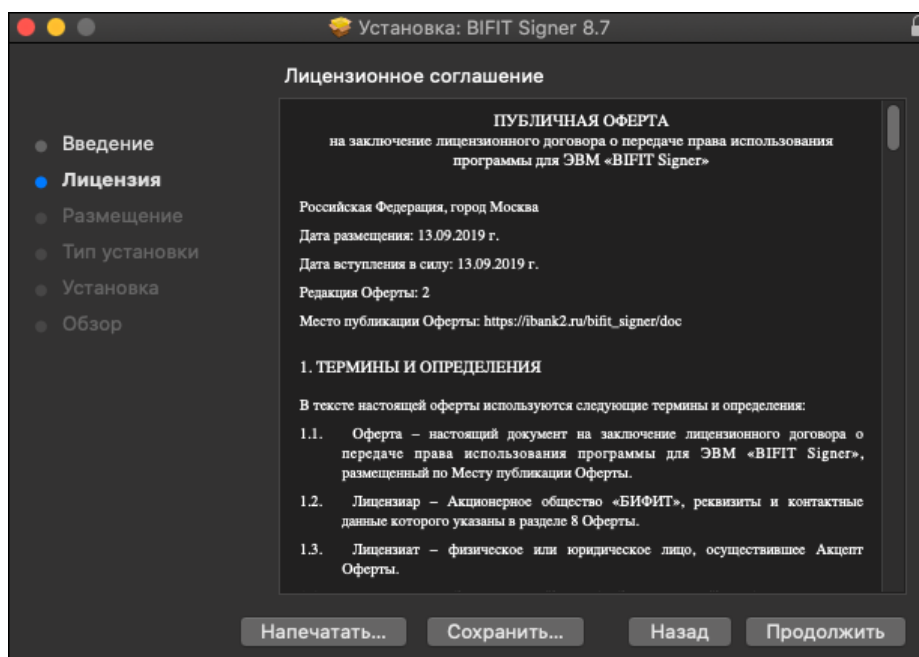
Рис. 8. Лицензионное соглашение
