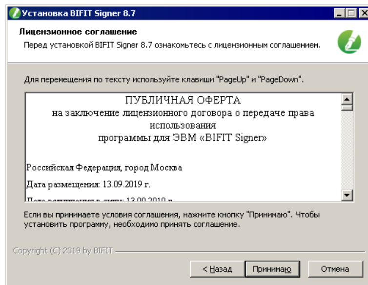
Рис. 4. Лицензионное соглашение
