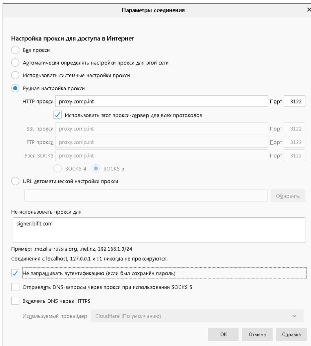
Рис. 21. Параметры соединения
