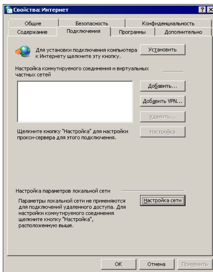
Рис. 18. Свойства браузера
