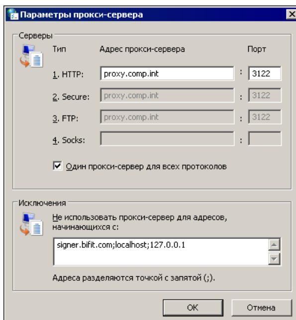
Рис. 20. Параметры прокси-сервера
